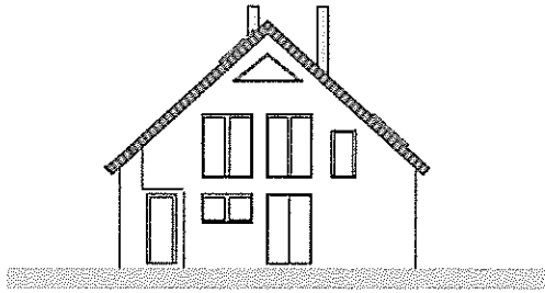
ansicht west
