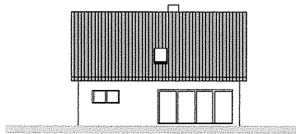
ansicht sud
